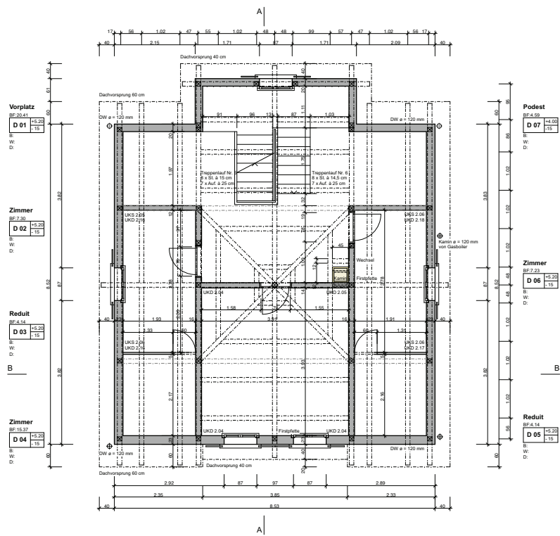
Grundriss Dachgeschoss
