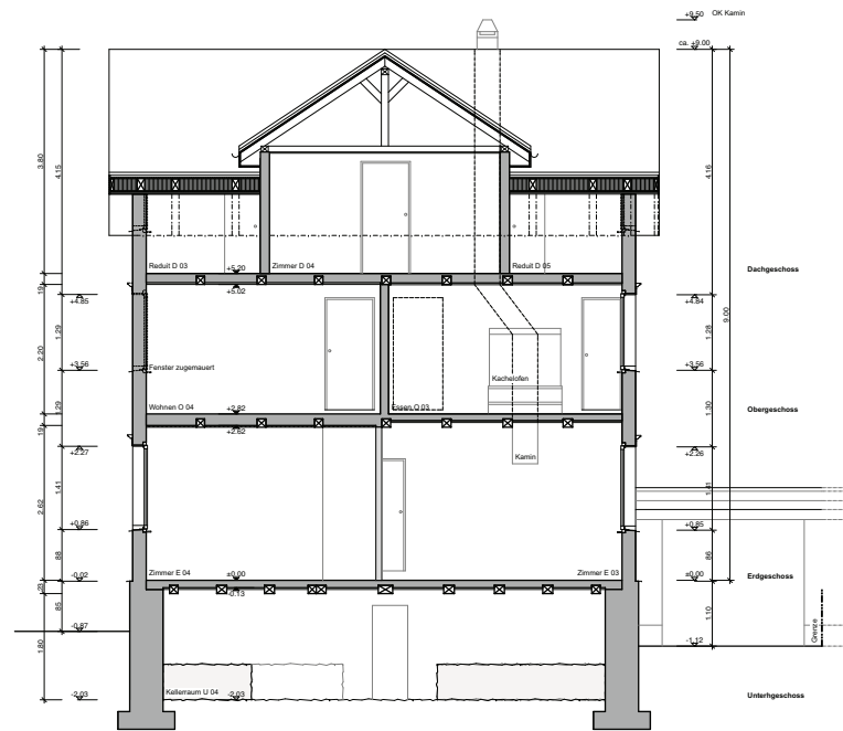
Schnitt BB
