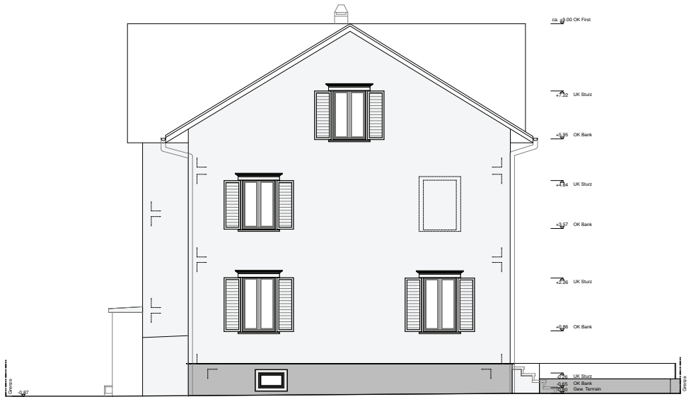
Ansicht Süd
