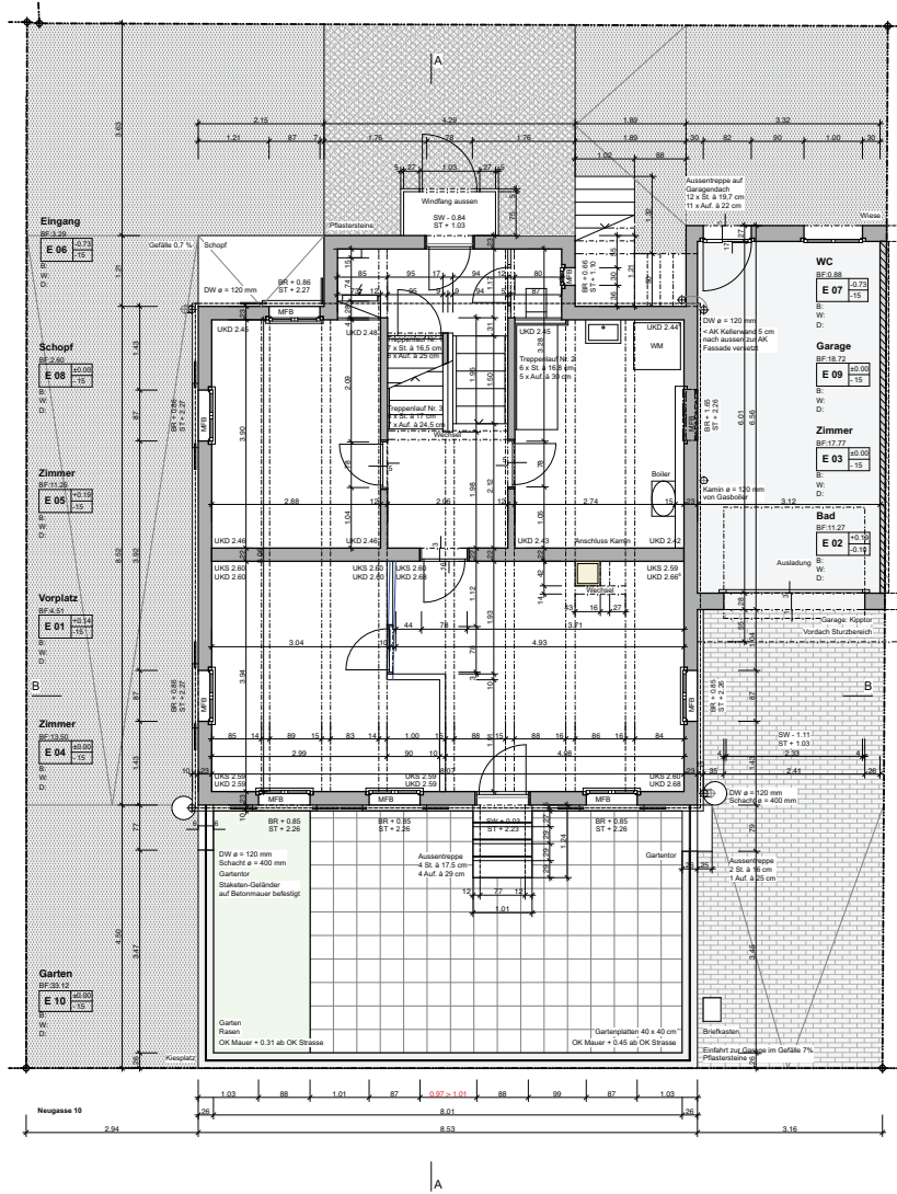
Grundriss Erdgeschoss
