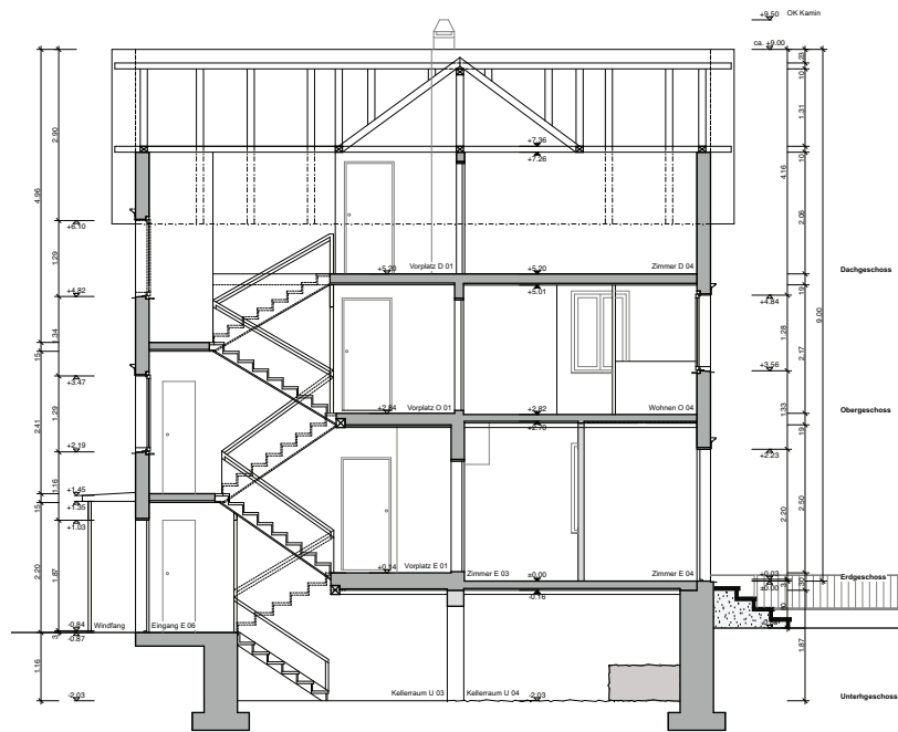
Schnitt AA
